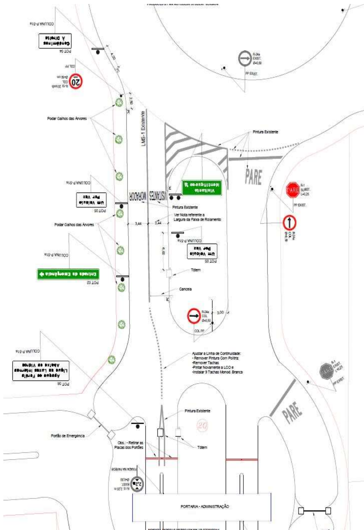
Parte do projeto de sinalização vertical
